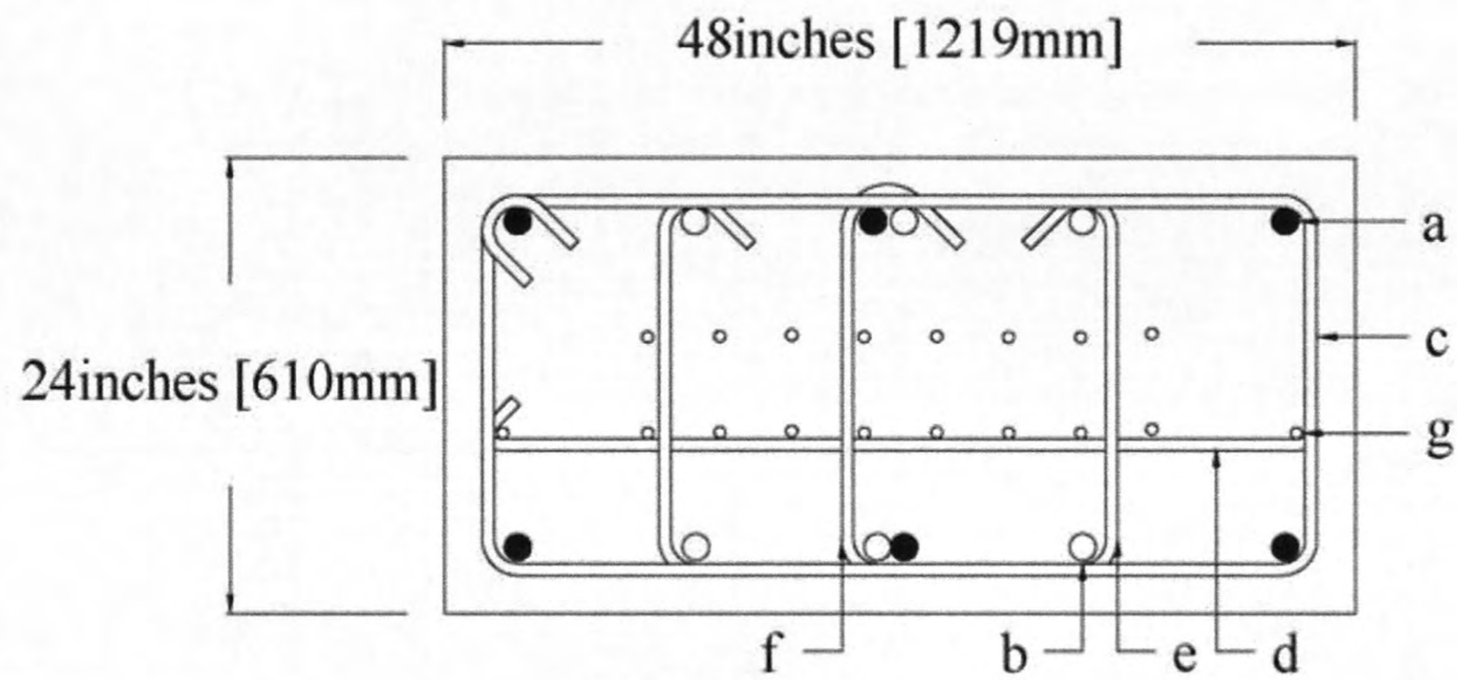
Section B-B End Region
