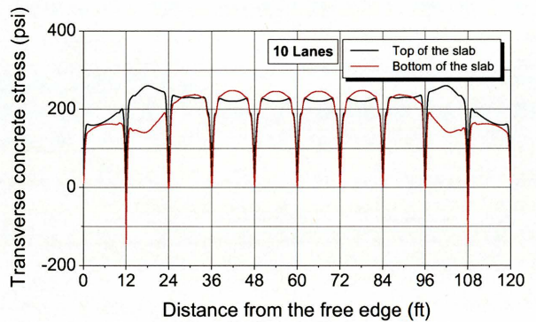
(d) Ten-lane pavement
