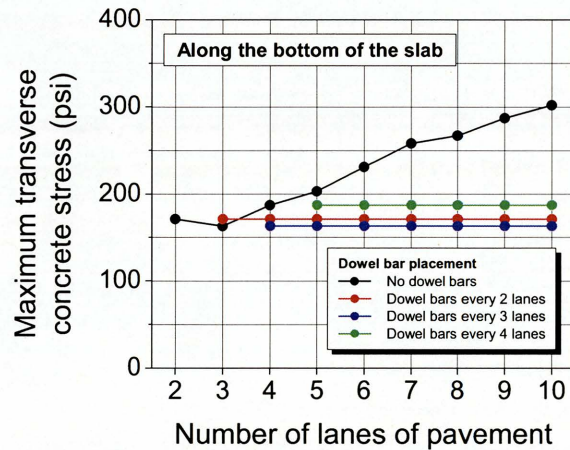
(d) Maximum concrete stress at the bottom of the slab
